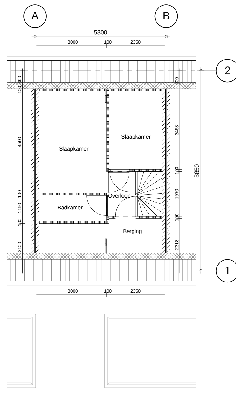
Verdieping - bestaand -
