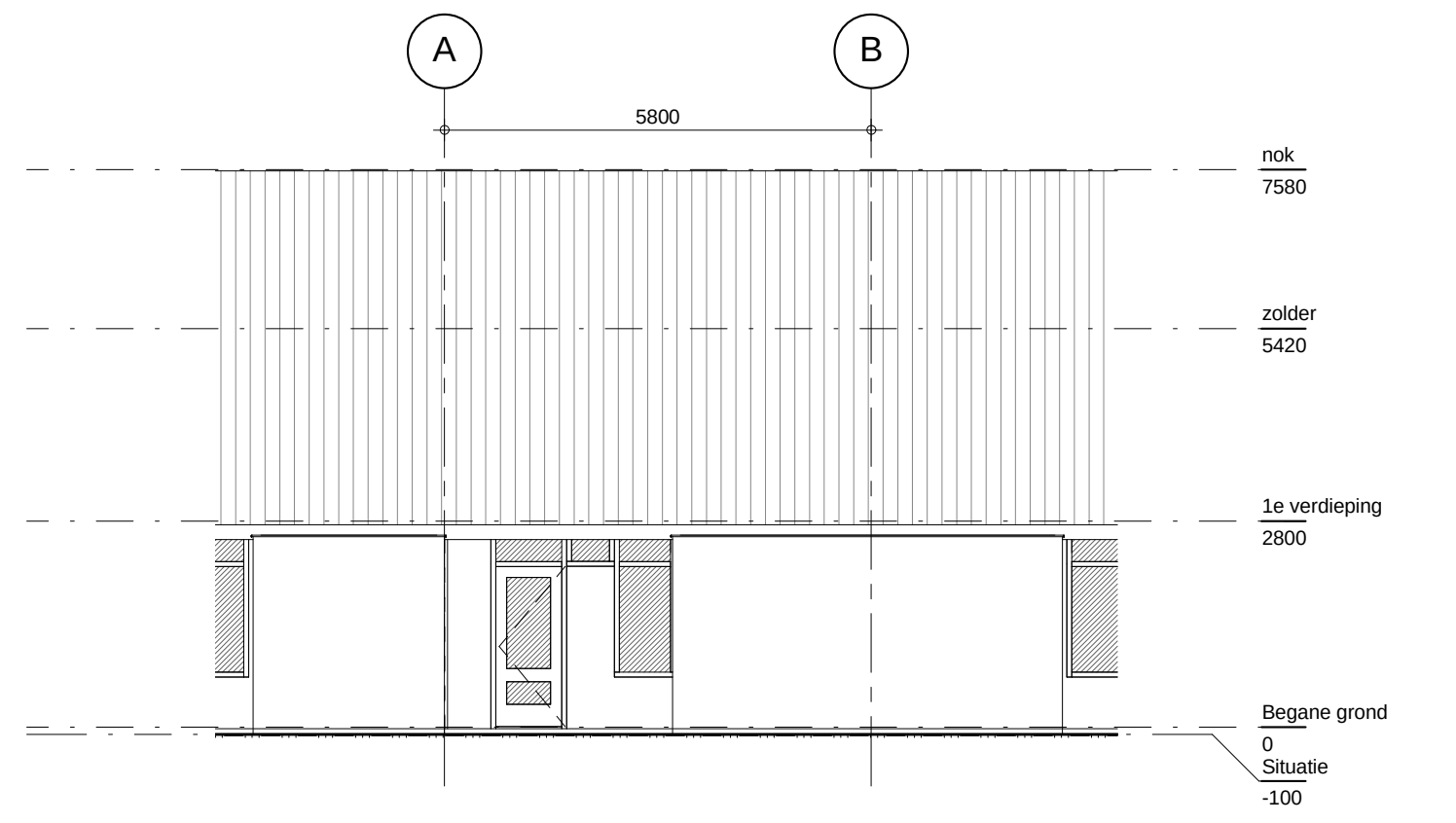
Voorgevel - bestaand -
