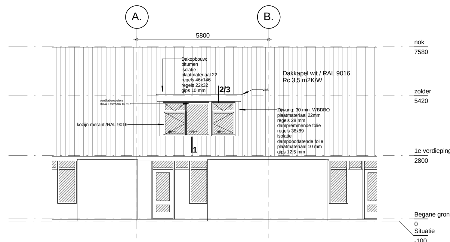
Voorgevel - nieuw -
