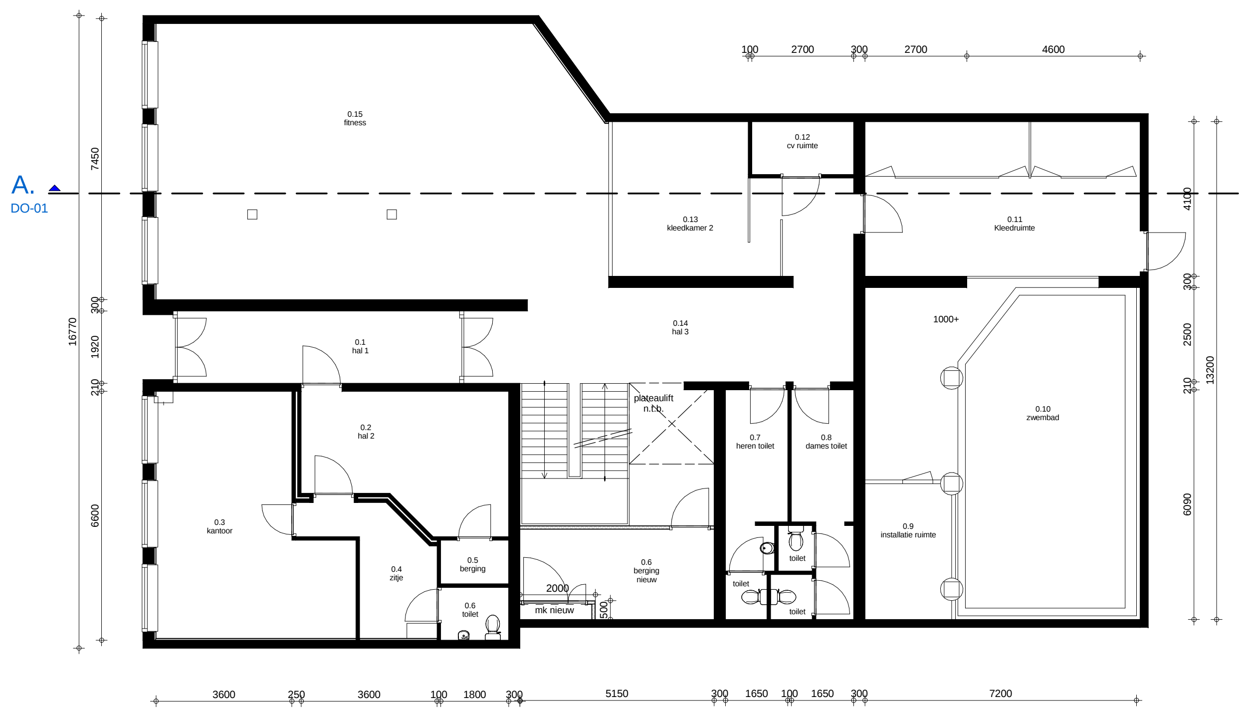
Begane grond - bestaand - schaal 1 : 100
