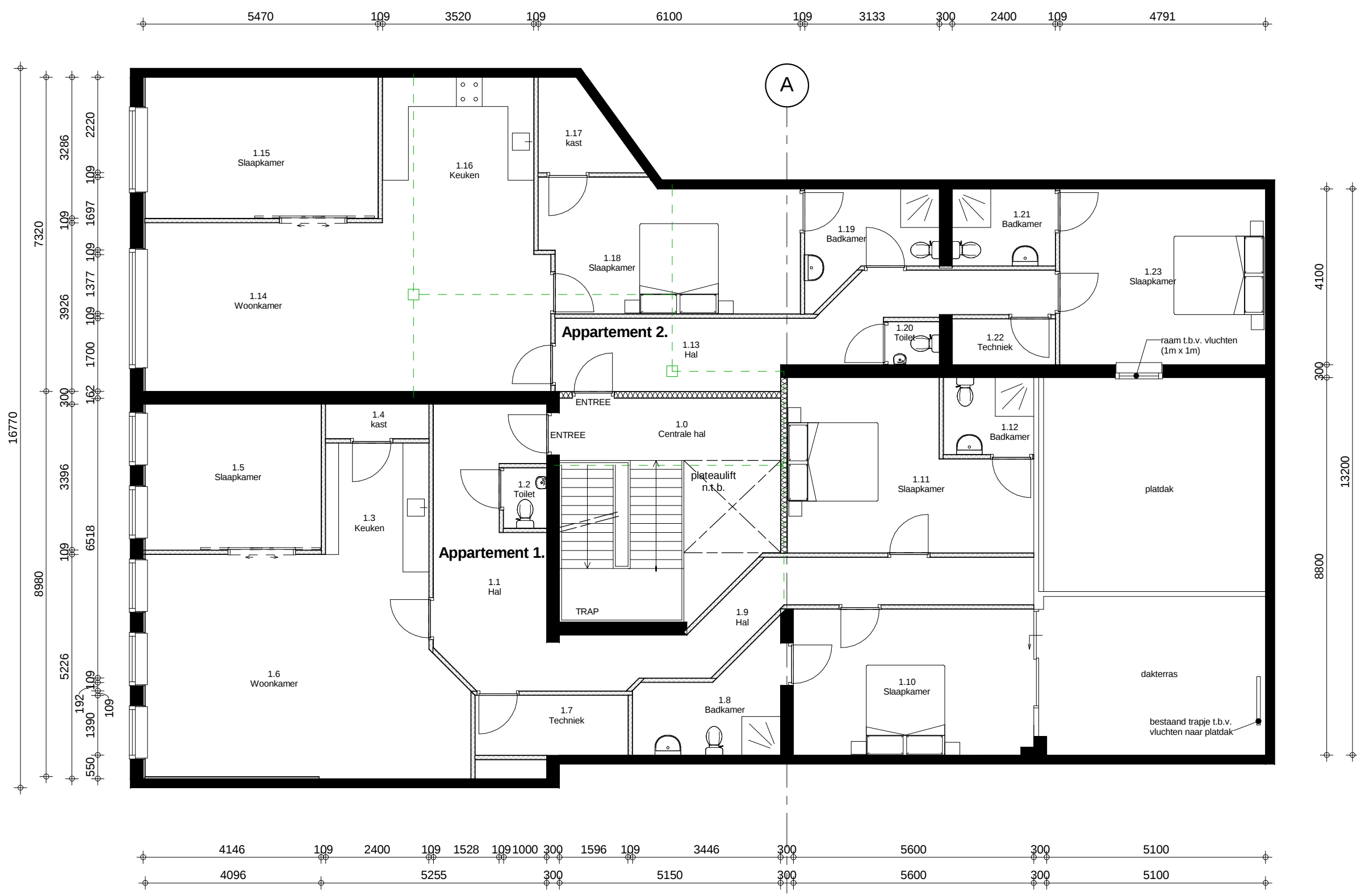
1e verdieping - nieuw - schaal 1 : 100
