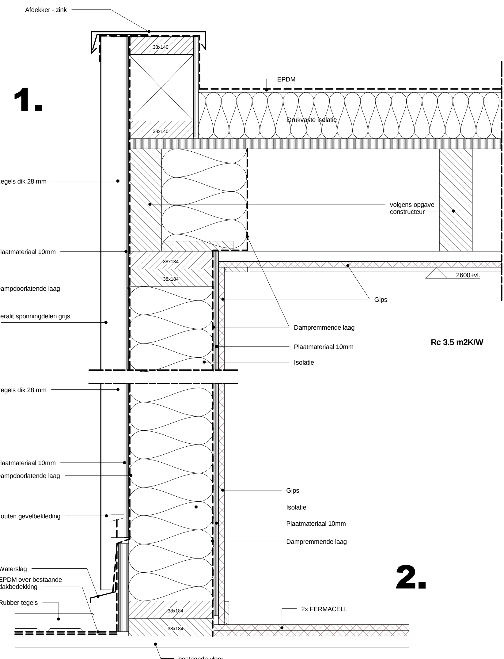
Details 1 en 2. schaal 1 : 5
