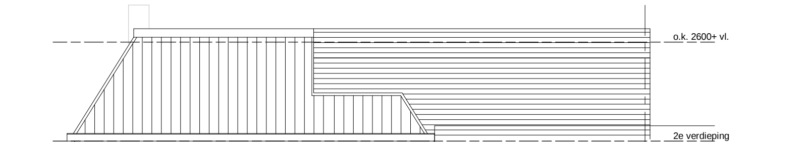
R.zijgevel - nieuw - schaal 1 : 100
