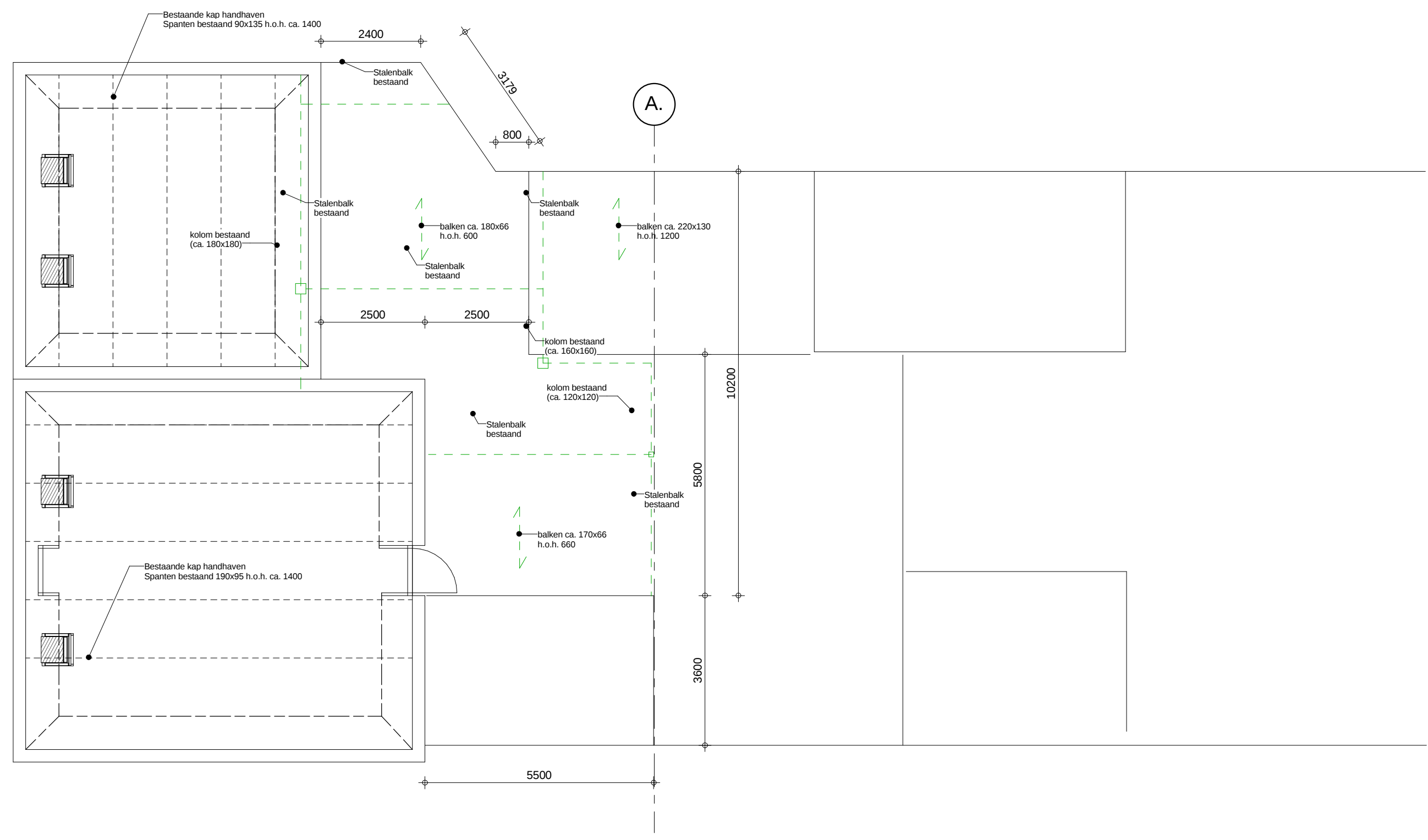
2e verdieping - bestaand - schaal 1 : 100
