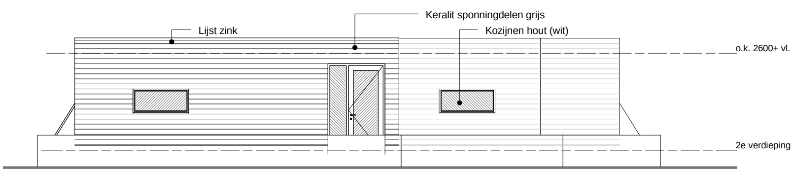
Achtergevel (dak) - nieuw - schaal 1 : 100
