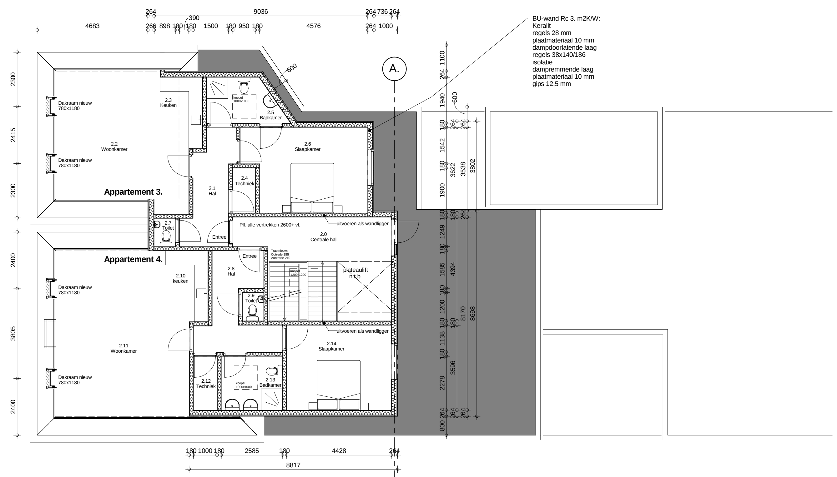
2e verdieping - nieuw - schaal 1 : 100
