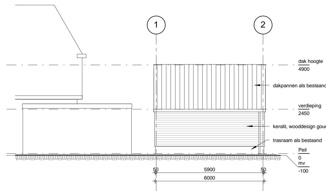
Rechterzijgevel hok
