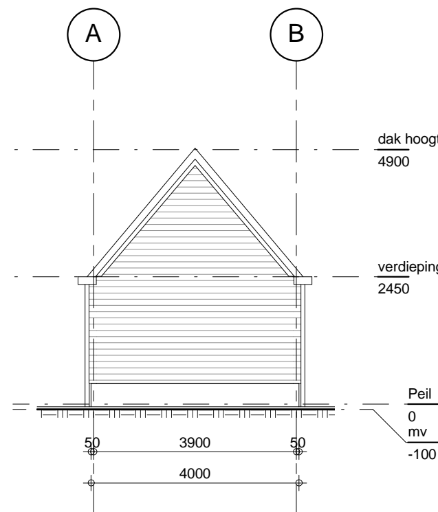
Achtergevel hok
