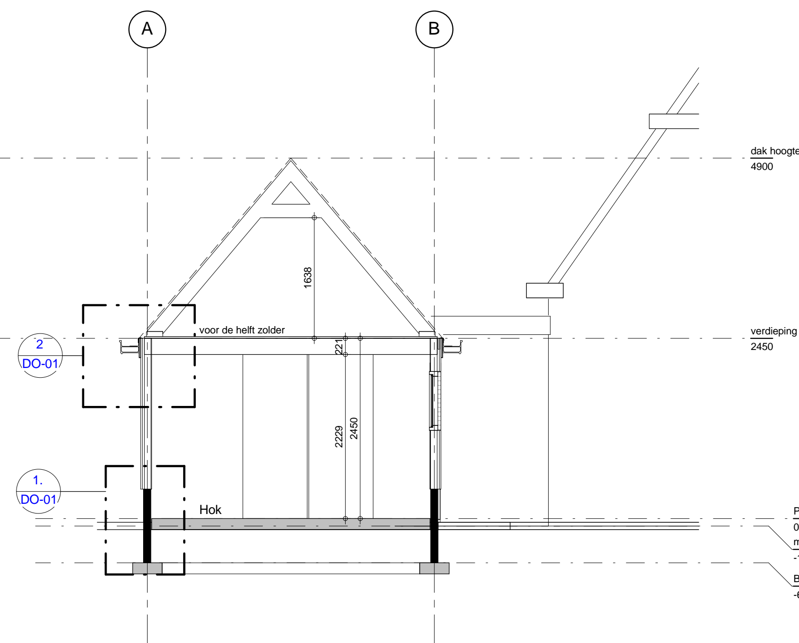
Doorsnede A-A
