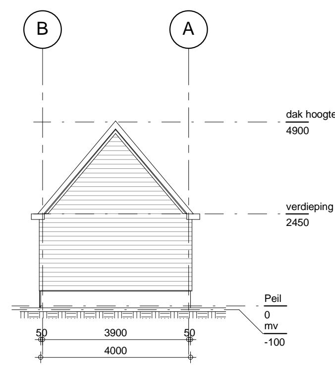
Voorgevel hok
