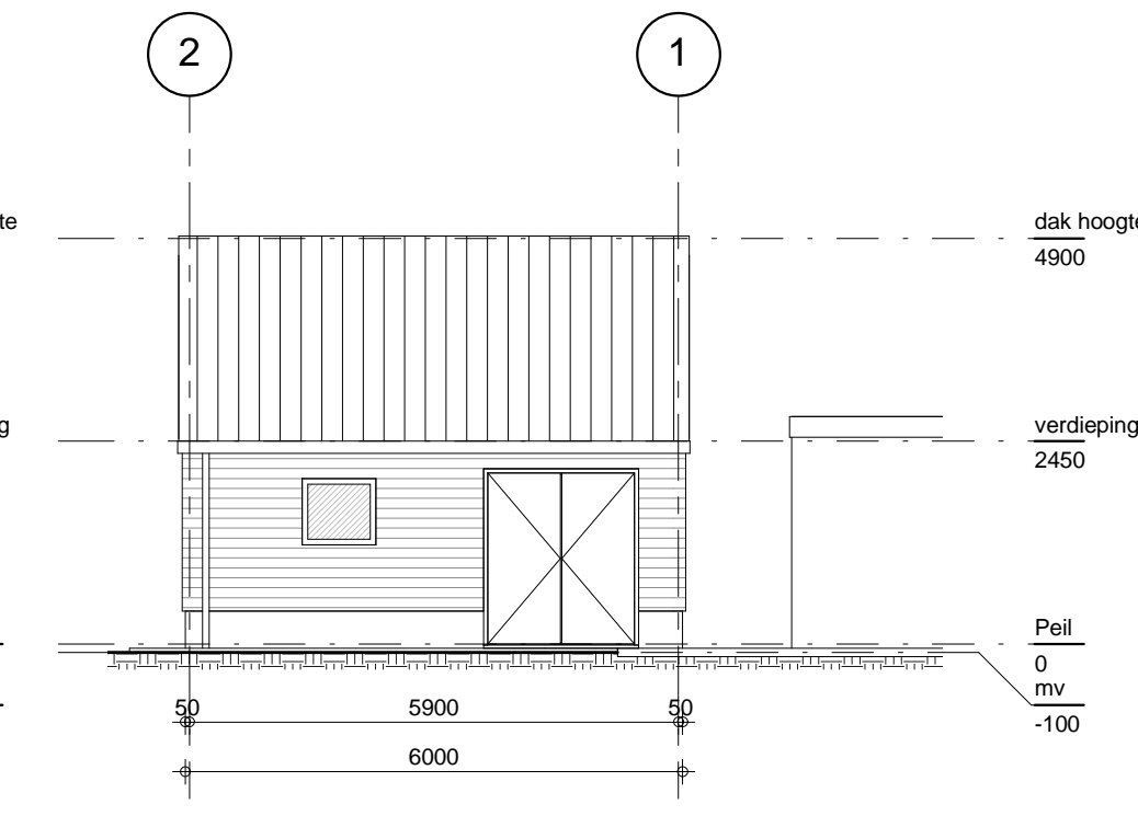
Linkerzijgevel hok
