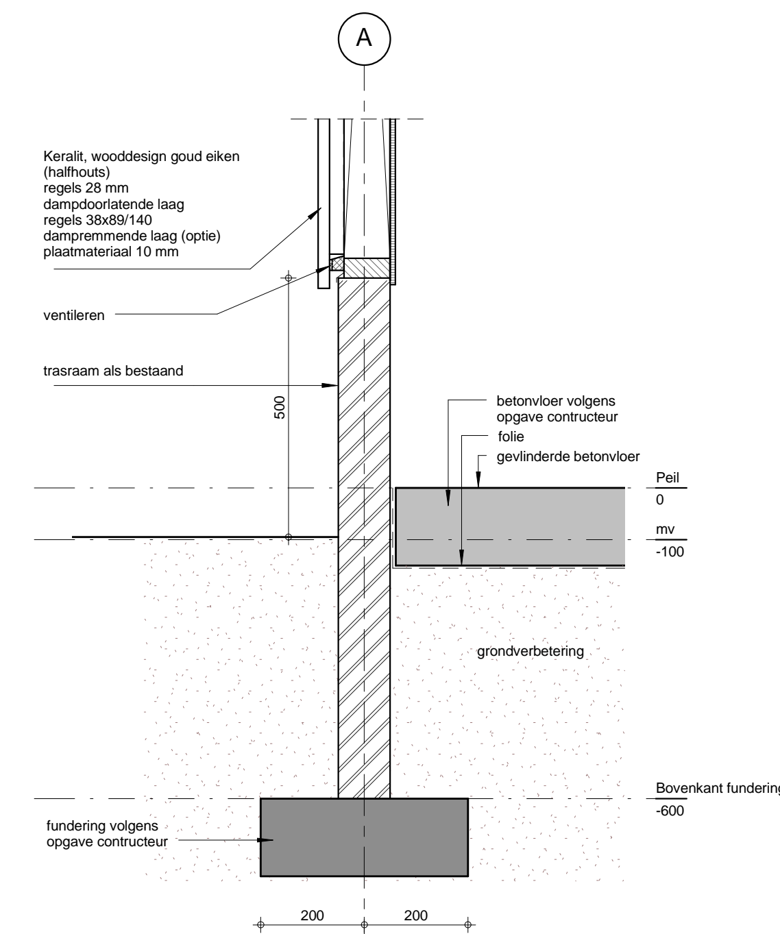
principe detail 1.
