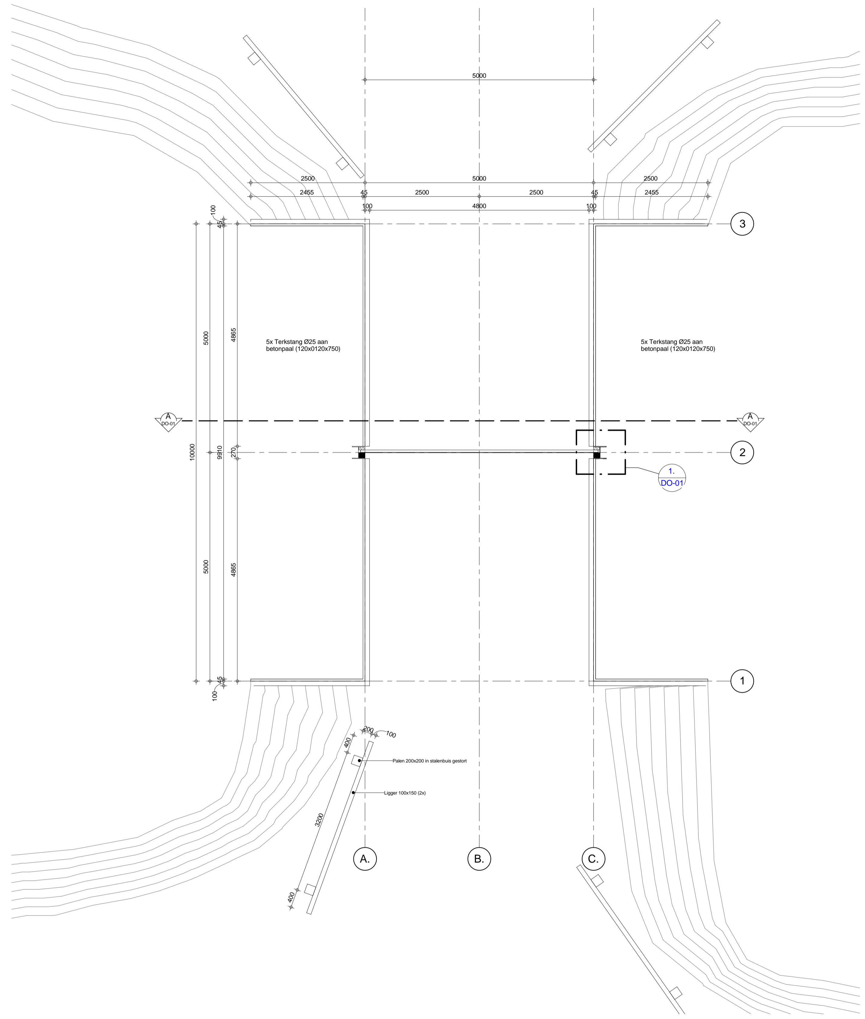
Boven aanzicht schaal 1 : 50
