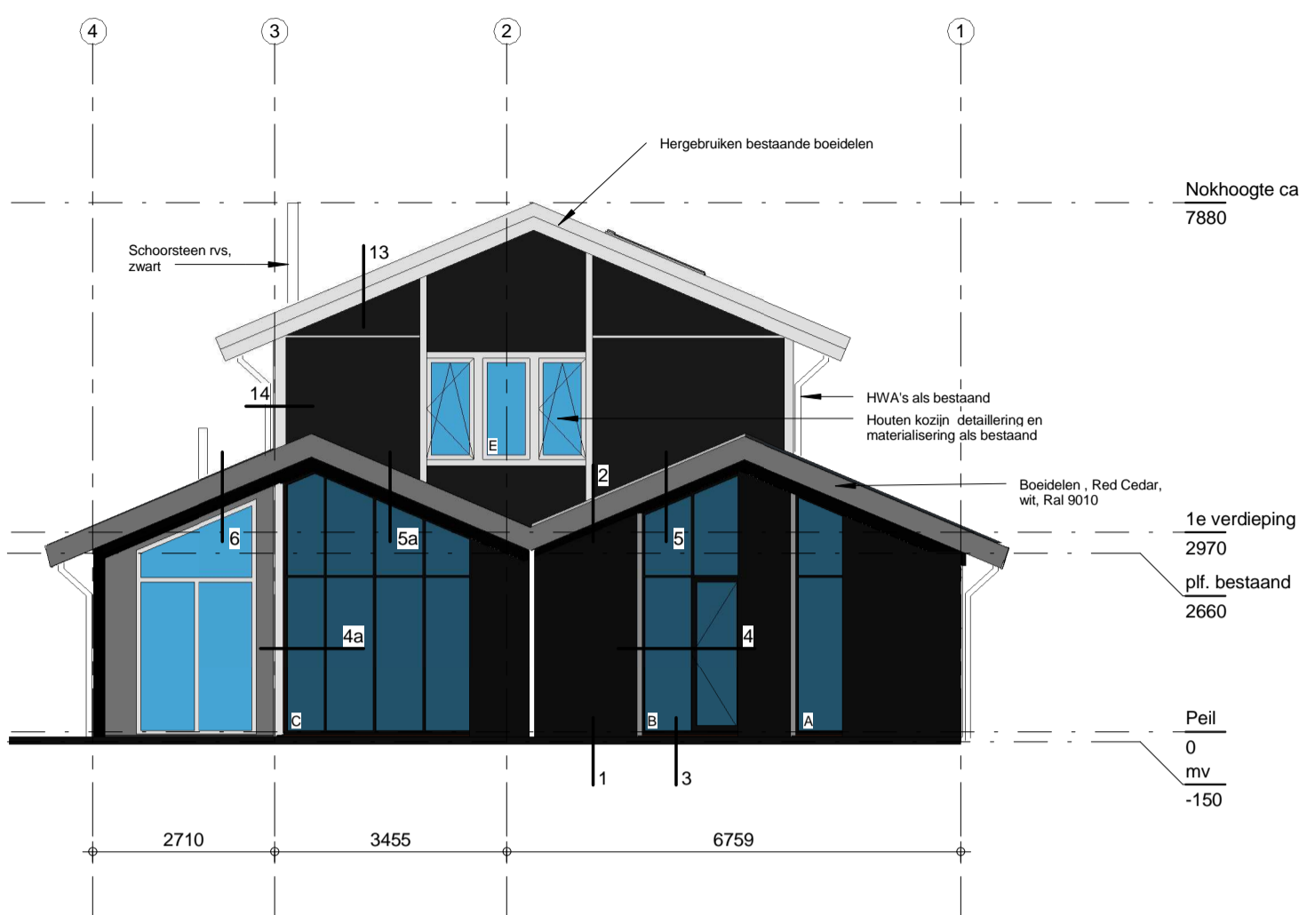
Oostgevel
