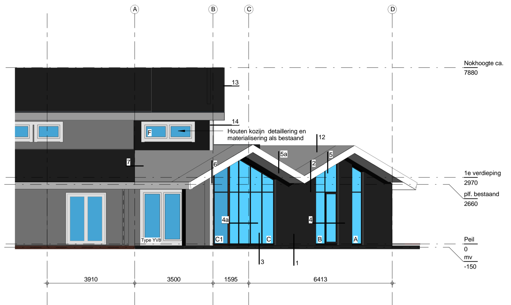
Zuidgevel
