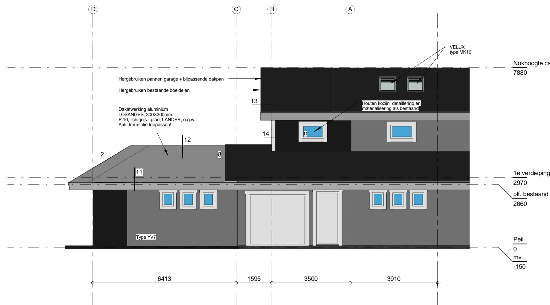
Noordgevel
