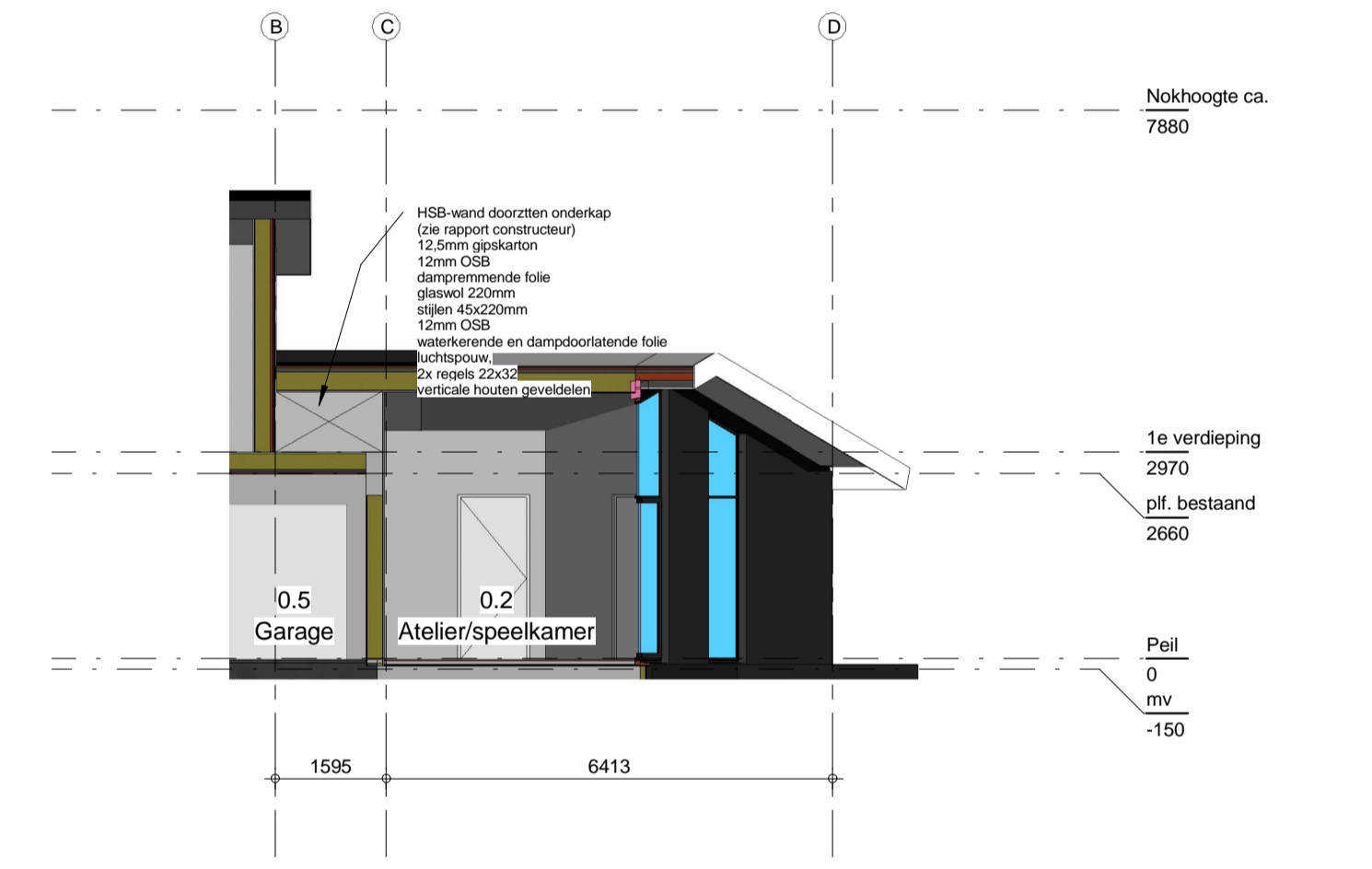
B-B
