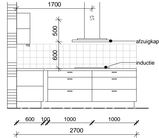
AANZICHT B
