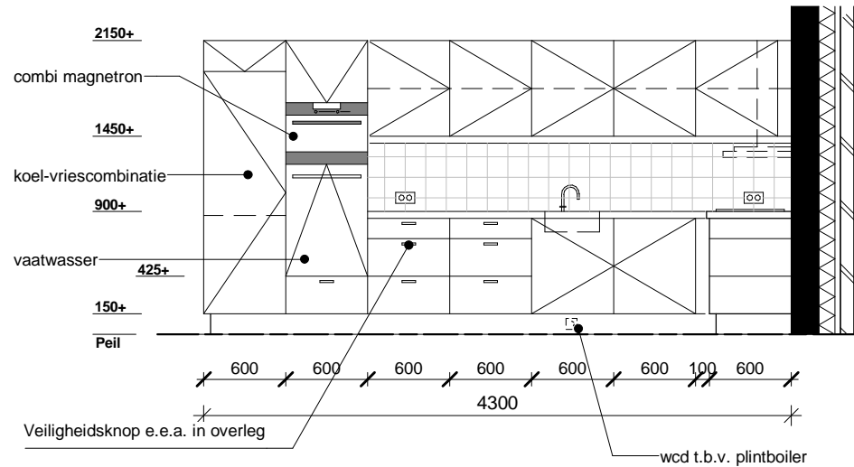
AANZICHT A
