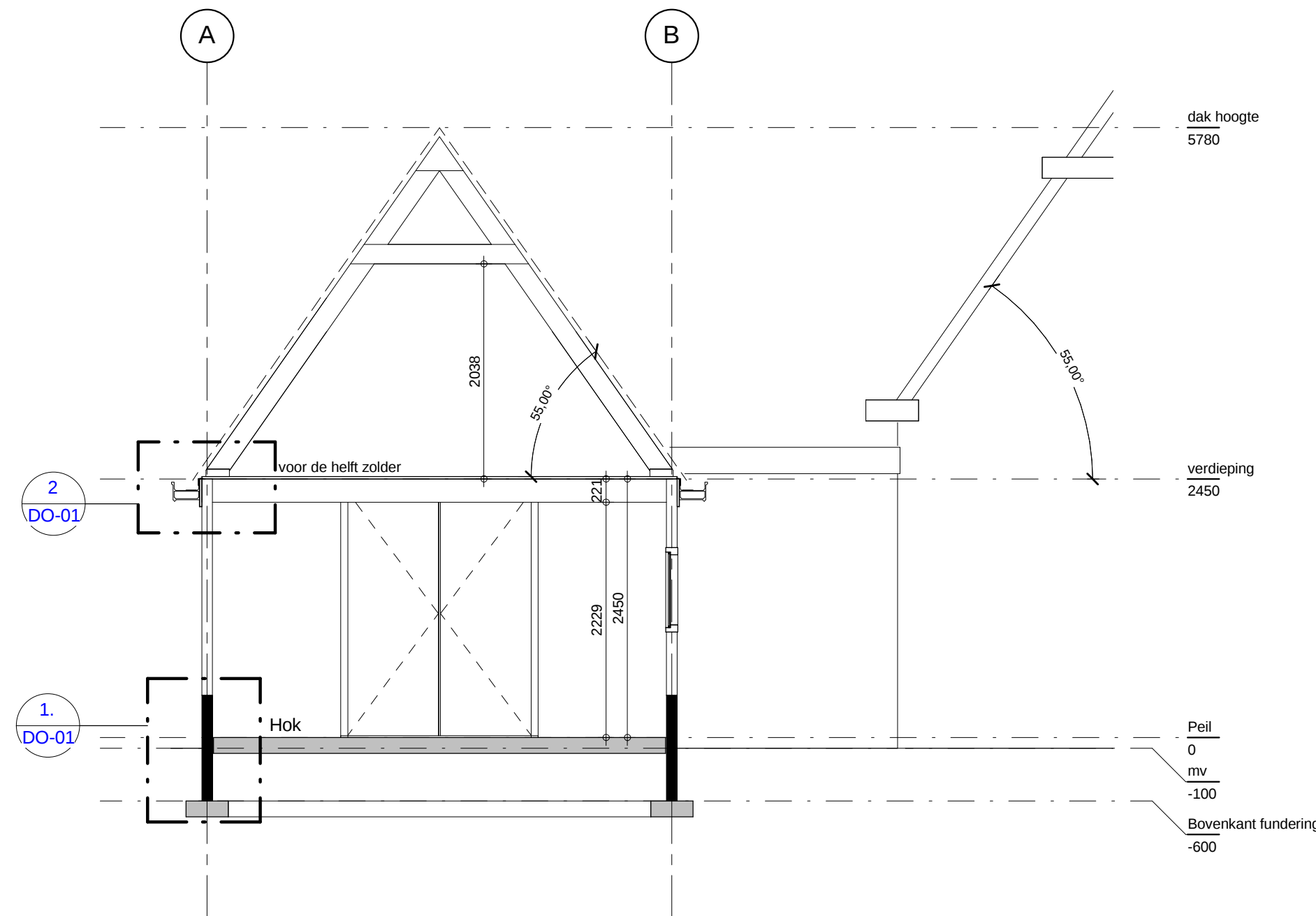
Doorsnede A-A
