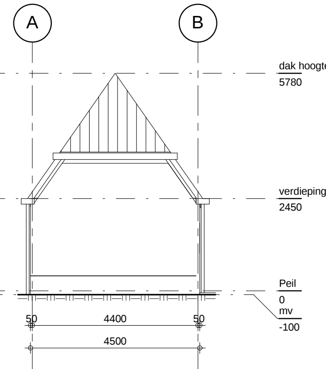
Achtergevel hok
