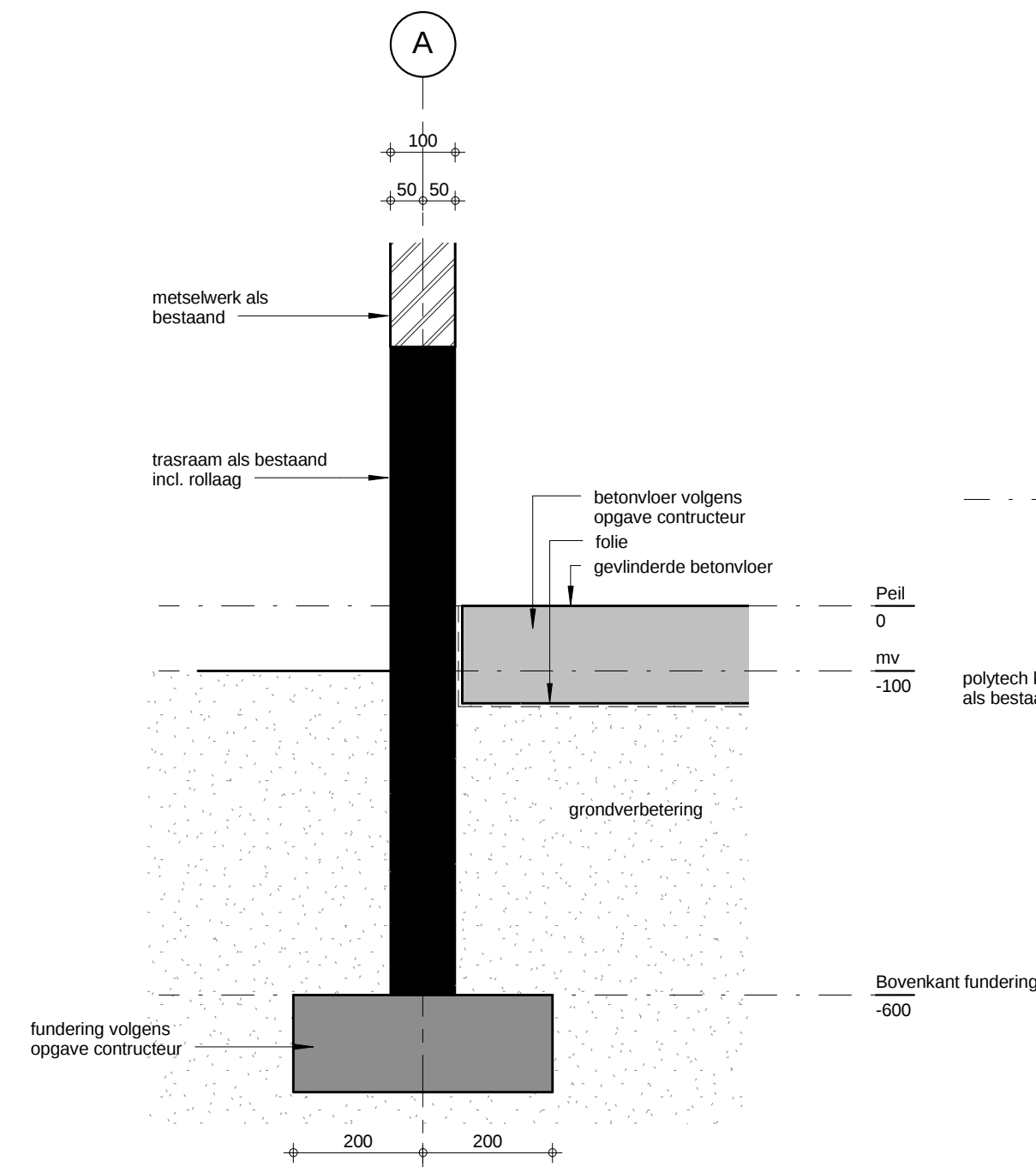
principe detail 1.
