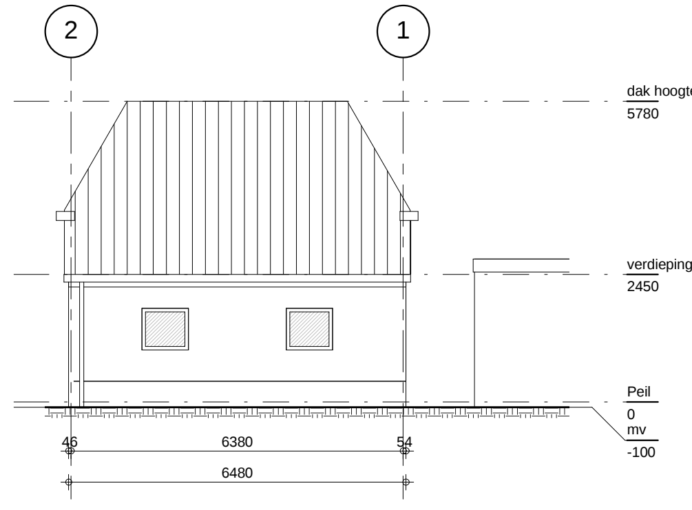
Linkerzijgevel hok
