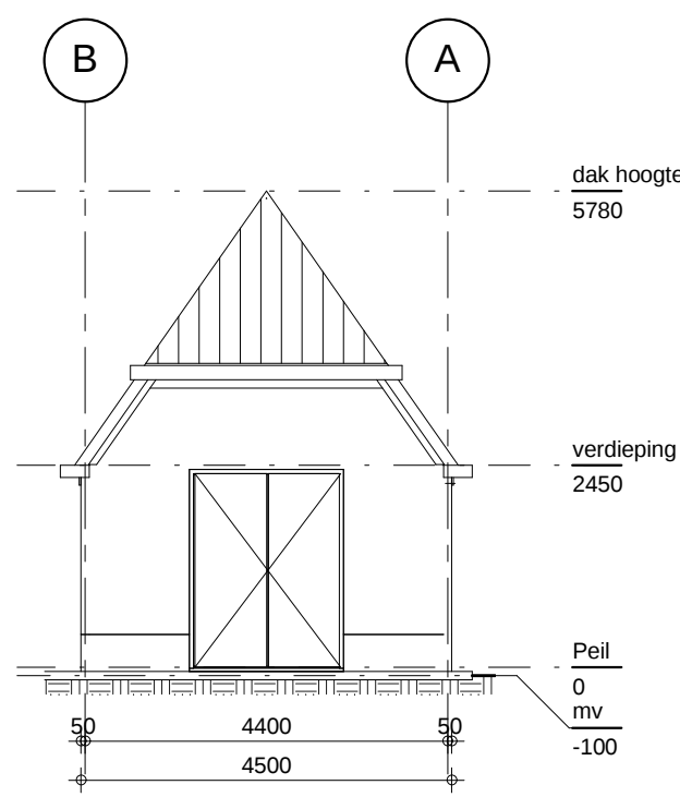
Voorgevel hok
