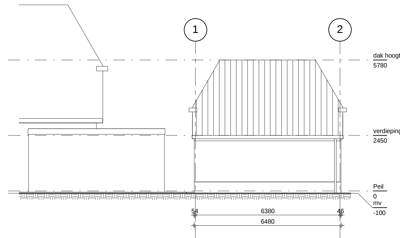
Rechterzijgevel hok
